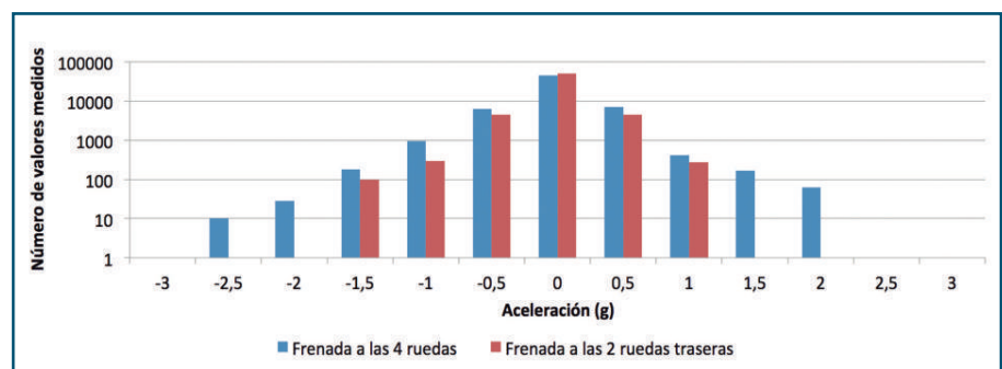
CUADRO IV. Prueba de maniobrabilidad.
